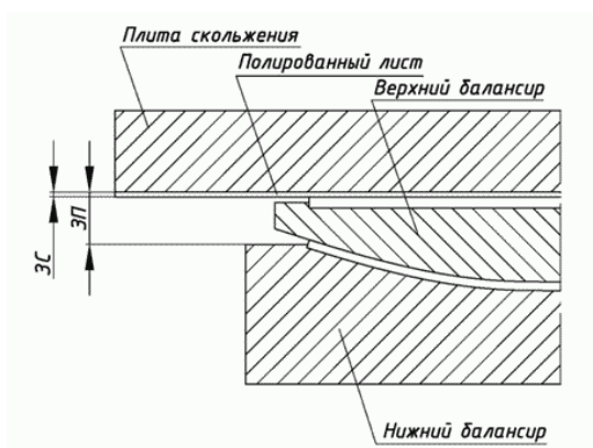
Рисунок 5. Схема измерения зазоров на сферических опорных частях
