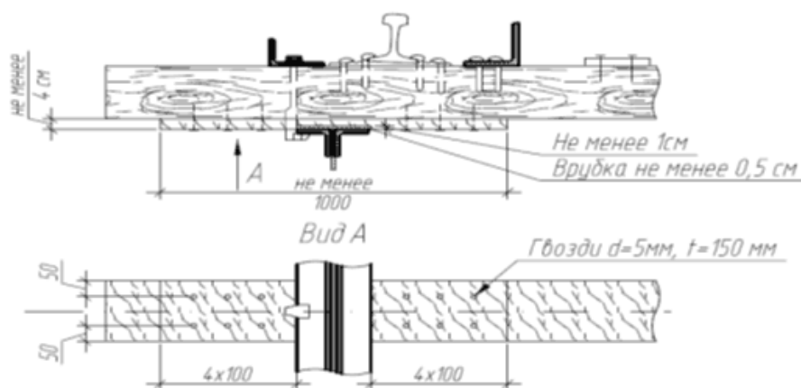
Рисунок 4. Увеличение высоты мостового бруса с помощью дополнительной доски
