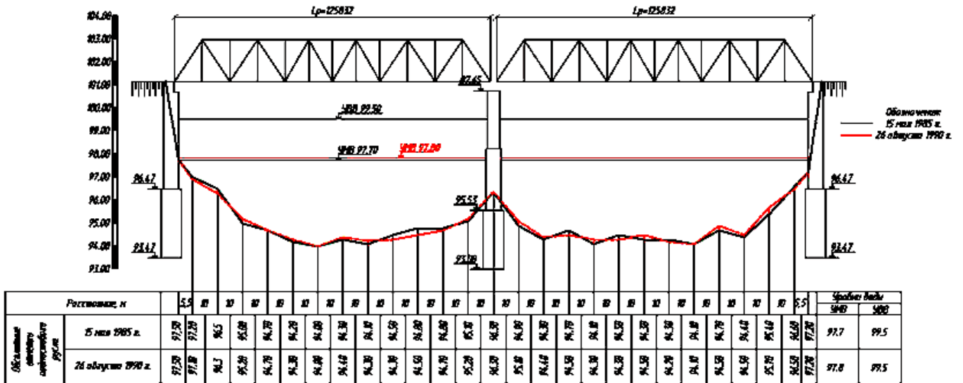
Рисунок 1. Поперечный профиль живого сечения реки
