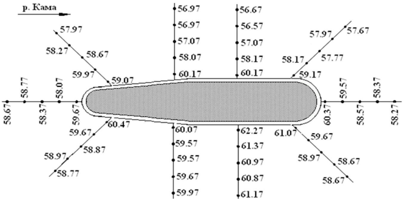
Рисунок 2. Результаты промеров глубин у опоры моста
