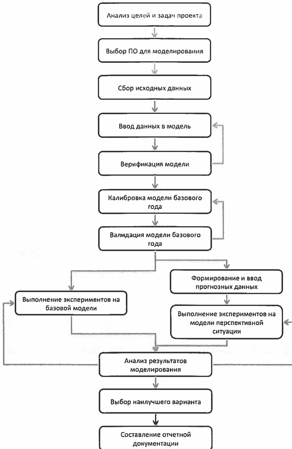
Рисунок 1 – Блок-схема процесса построения модели участка УДС
