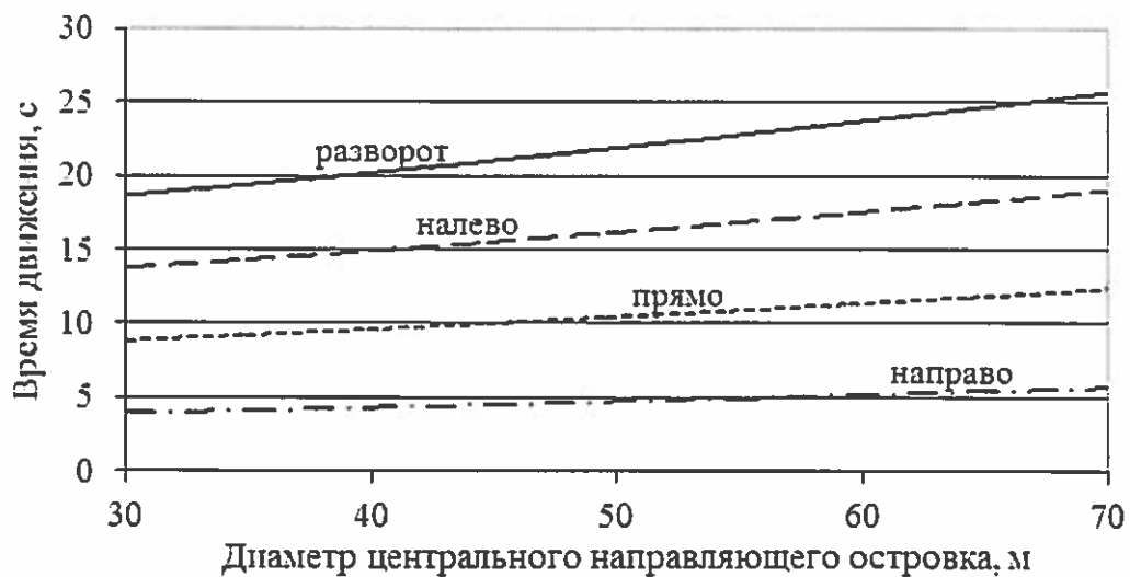
Рисунок 2.20 - Зависимость геометрической задержки транспортного средства от диаметра центрального направляющего островка
