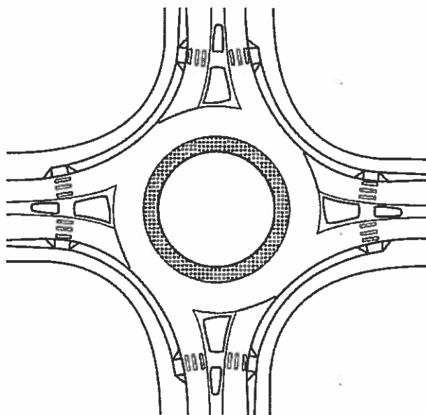
Рисунок 1.17 – Планировка малого кольцевого пересечения (пример)
