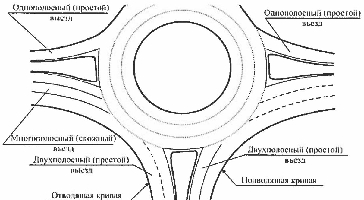
Рисунок 1.5 - Виды въездов (выездов) кольцевых пересечений
