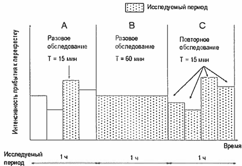
Рисунок 3.3 – Методы измерения пиковой интенсивности движения
