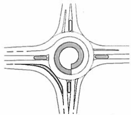
б) Пропускная способность 3500 ед/ч
