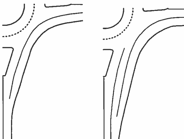
Рисунок 1.16 - Варианты размещения специальных правоповоротных полос
