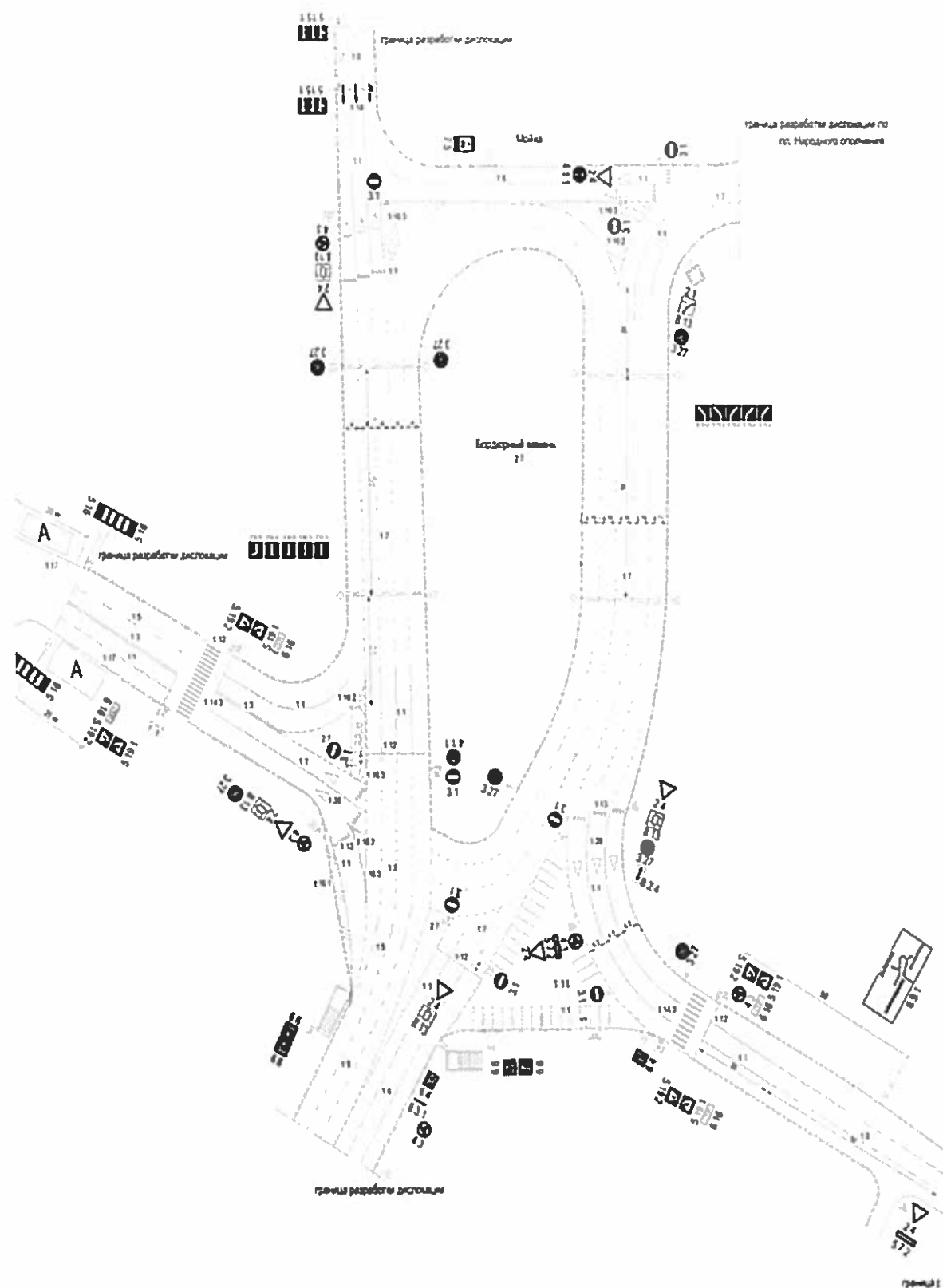
Рисунок 2.25 – Пример применения технических средств организации движения на площади с элементами кругового движения
