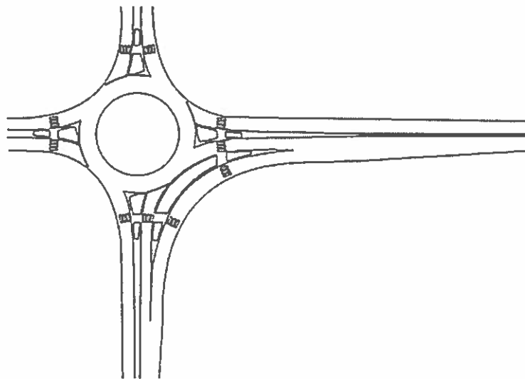
Рисунок 1.14 - Кольцевое пересечение со специальной правоповоротной полосой и переходно-скоростной полосой
