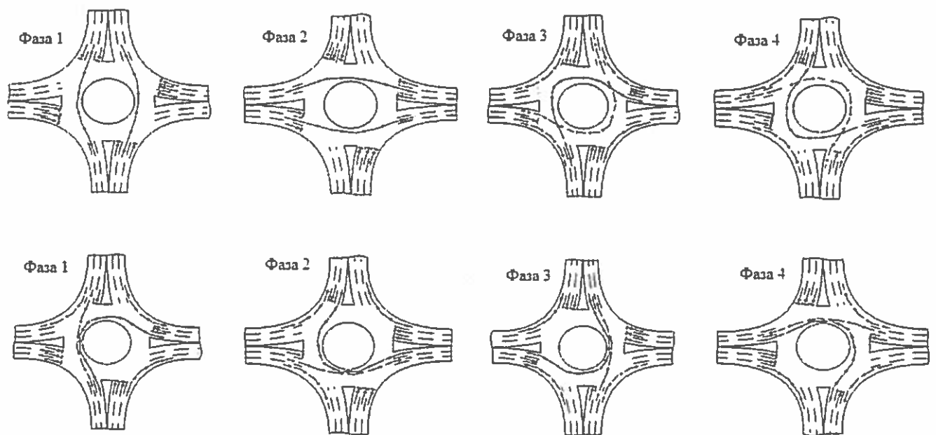
Рисунок 2.19 – Метод организации светофорного регулирования «Смешанный»
