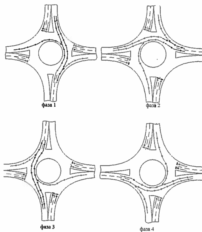
Рисунок 2.17 - Метод организации светофорного регулирования «Зелёная турбина»
