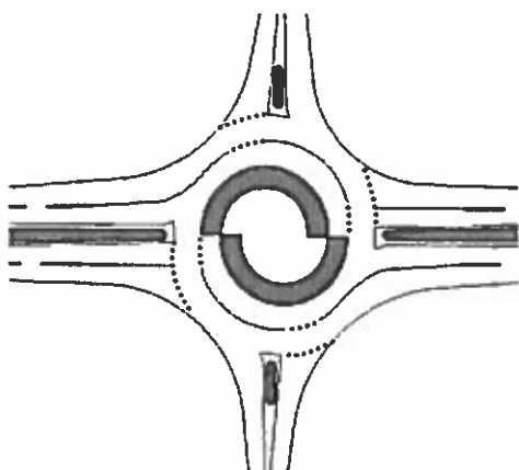
а) Пропускная способность 2800 ед/ч
