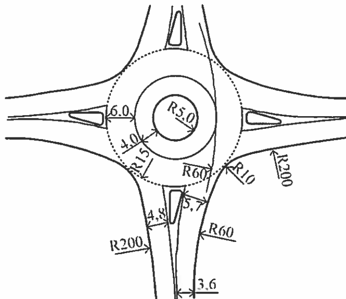
Рисунок 1.18 - План и параметры узла
