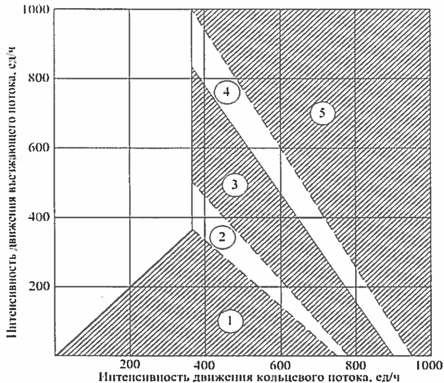
Рисунок 1.21 - Пределы эффективного применения малых кольцевых пересечений
