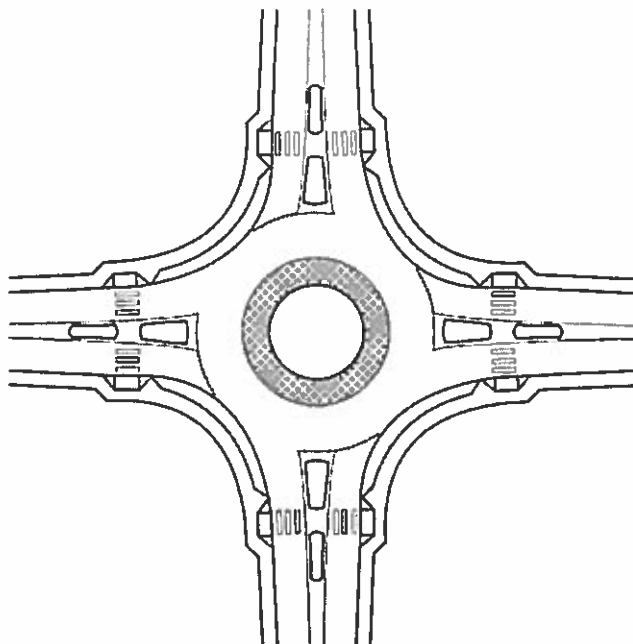
Рисунок 1.20 - План и параметры узла с объезжаемым островком
