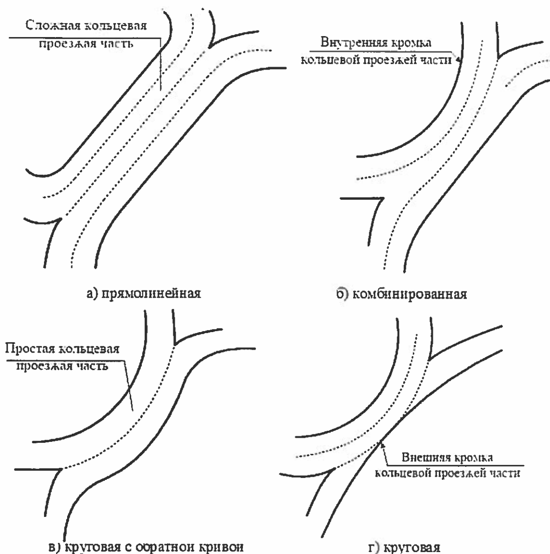
Рисунок 1.12 - Формы и виды кольцевой проезжей части
