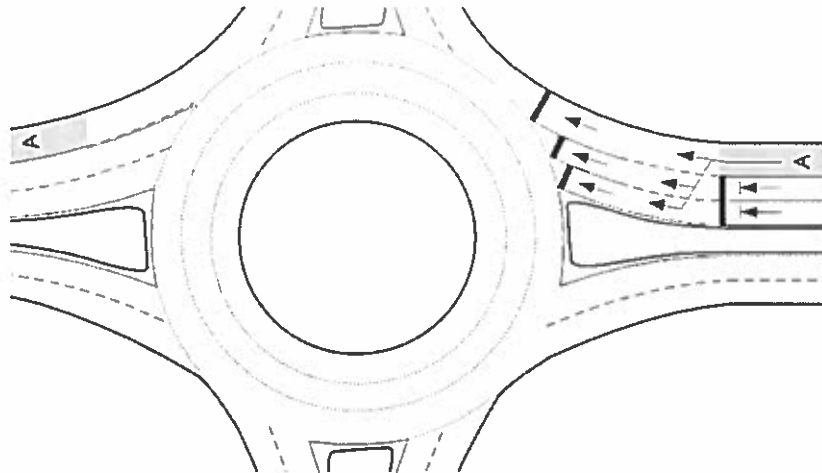
Рисунок 2.13 - Организация приоритетного проезда пересечения методом разнесённых стоп-линий
