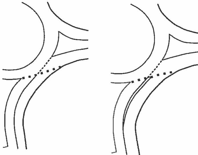
Рисунок 1.13 - Варианты устройства специальных правоповоротных полос
