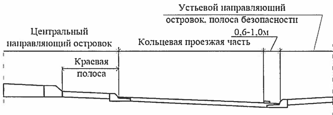
Рисунок 1.19 - Параметры и схема устройства краевых полос
