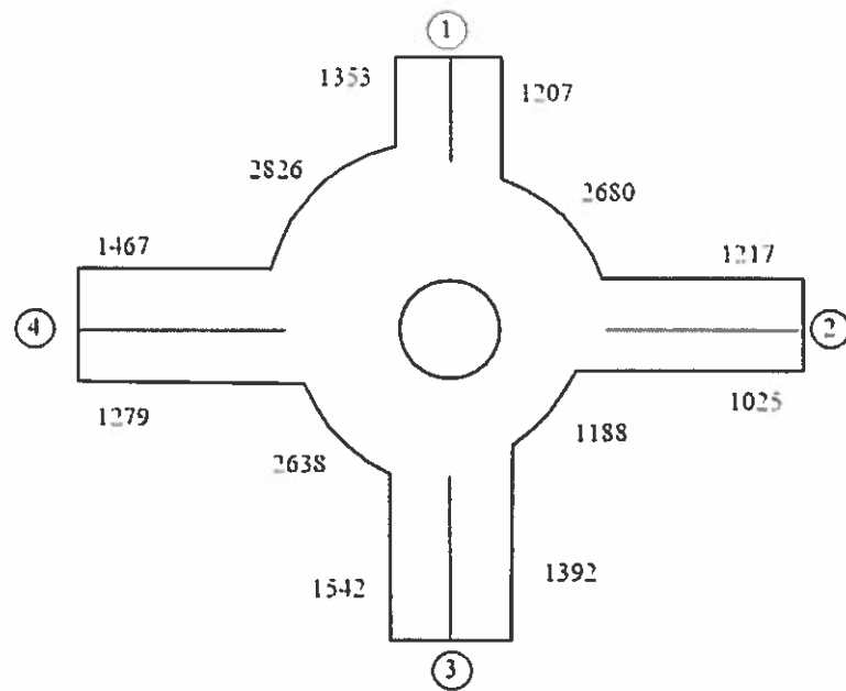
Рисунок 3.6 - Вид эпюры интенсивности движения на кольцевом пересечении
