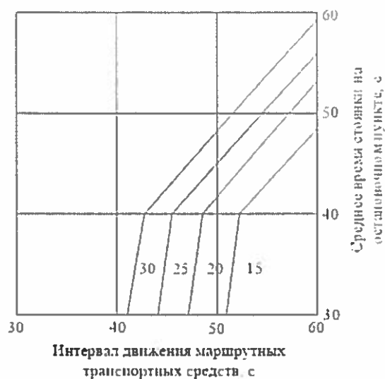
Рисунок 2.7 - Номограмма выбора расстояния удаления остановочного пункта (с одним местом для маршрутных транспортных средств)
