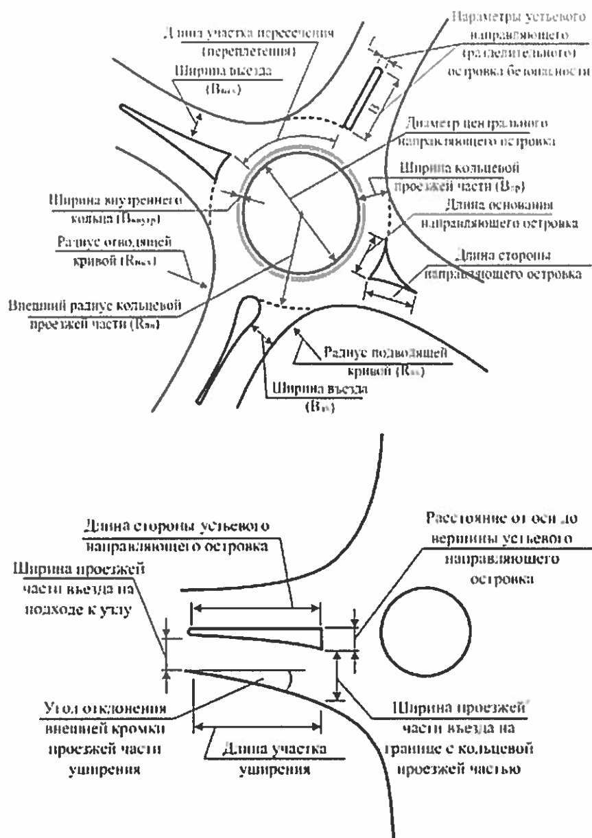
Рисунок 1.2 - Геометрические параметры элементов кольцевых пересечений
