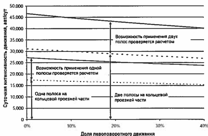
Рисунок 1.1 – Предварительный выбор количества полос движения на кольцевой проезжей части для мини-кольцевых пересечений, кольцевых пересечений малого и среднего диаметра
