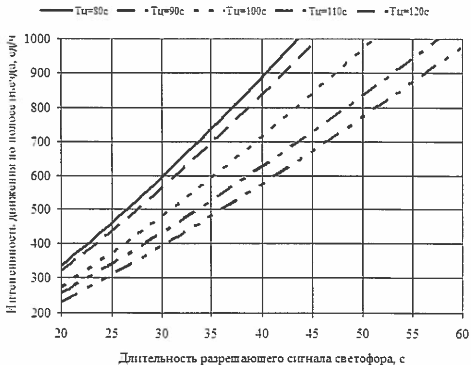
Рисунок 2.21 - Номограмма выбора длительности основного такта
