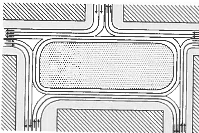
Рисунок 1.24 - Площадь с круговым движением
