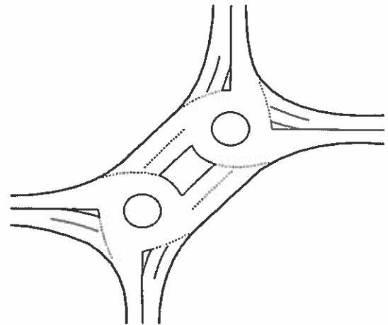
Рисунок 1.29 - Пересечения канализированного типа со сложной планировкой и элементами кругового движения
