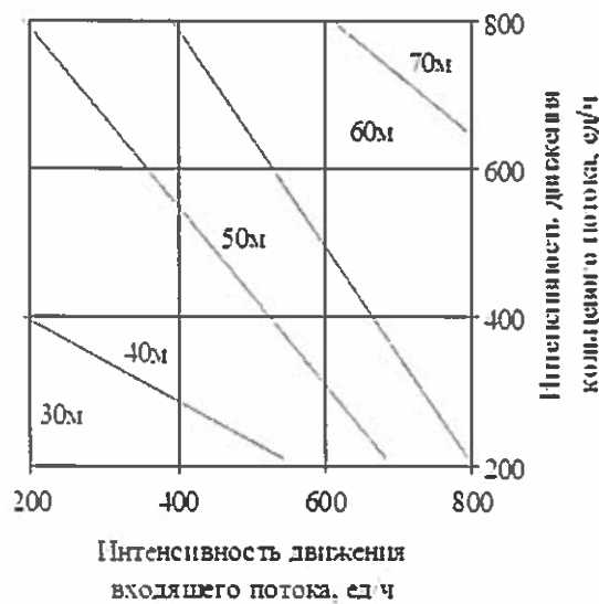
Рисунок 1.11 - Номограмма выбора минимально необходимой длины участка переплетения при расчётной скорости движения 40 км/ч
