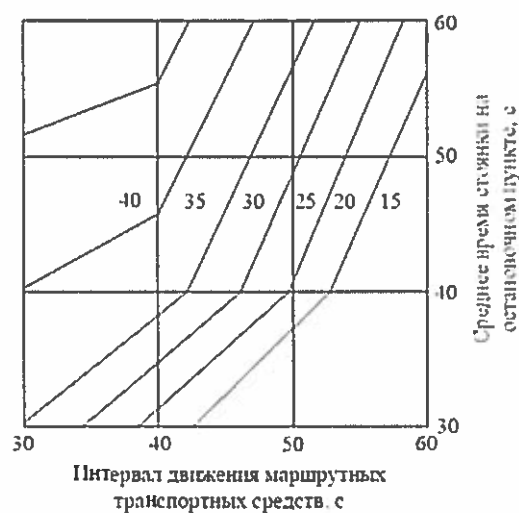
Рисунок 2.9 - Номограмма выбора расстояния удаления остановочного пункта (с тремя местами для маршрутных транспортных средств)
