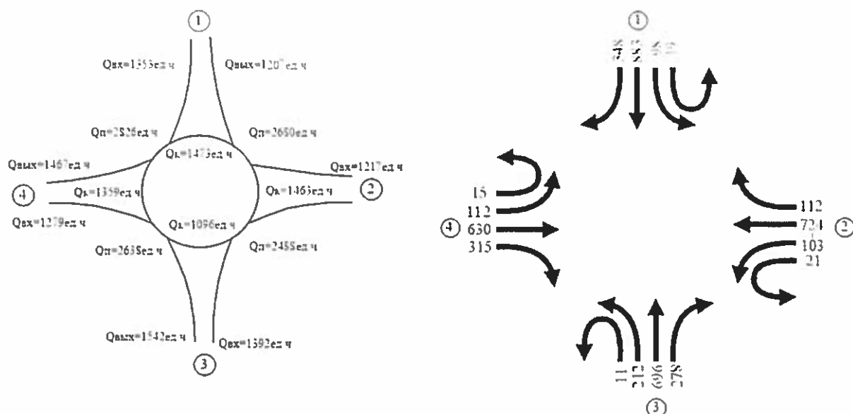
Рисунок 3.8 - Варианты цифрограмм интенсивности движения на кольцевом пересечении
