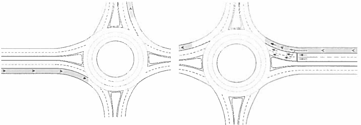
Рисунок 2.10 - Выделение приоритетной полосы по всей улице
