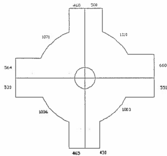
Рисунок 6.1 - Эпюра интенсивности движения в узле
