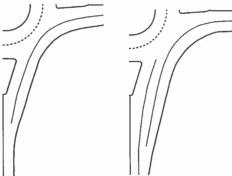
Рисунок 1.15 - Варианты размещения специальных правоповоротных полос
