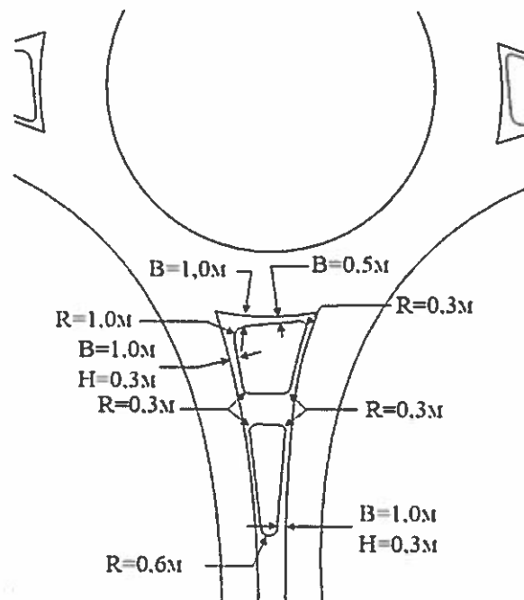
Рисунок 1.8 - Геометрические параметры устьевых направляющих островков
