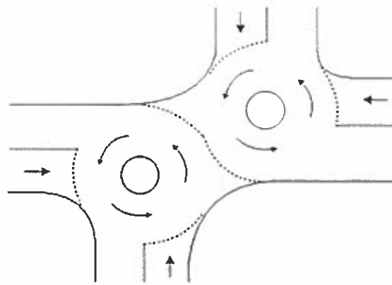
Рисунок 1.23 - Реализация круговой схемы движения на сдвинутом пересечении
