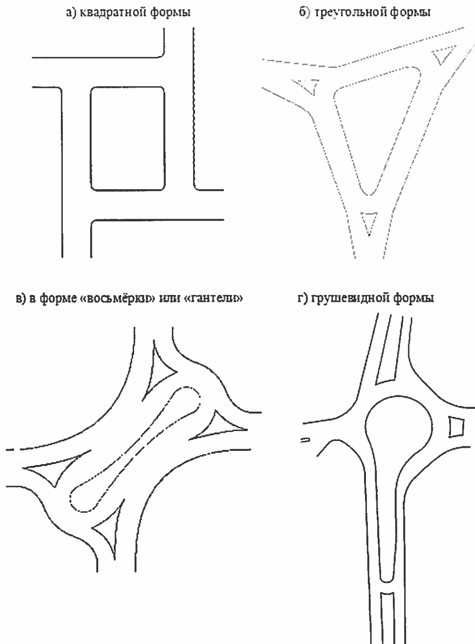
Рисунок 1.3 - Центральные направляющие островки нестандартной формы
