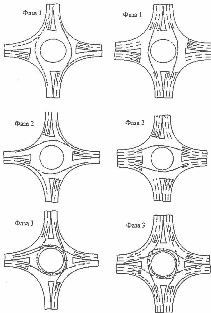
Рисунок 2.18 - Метод организации светофорного регулирования «Классический»
