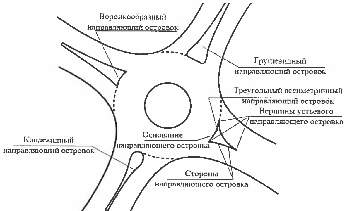
Рисунок 1.7 - Виды, формы и элементы устьевых направляющих островков
