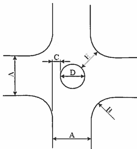
Рисунок 1.22 - Геометрические параметры пересечения
