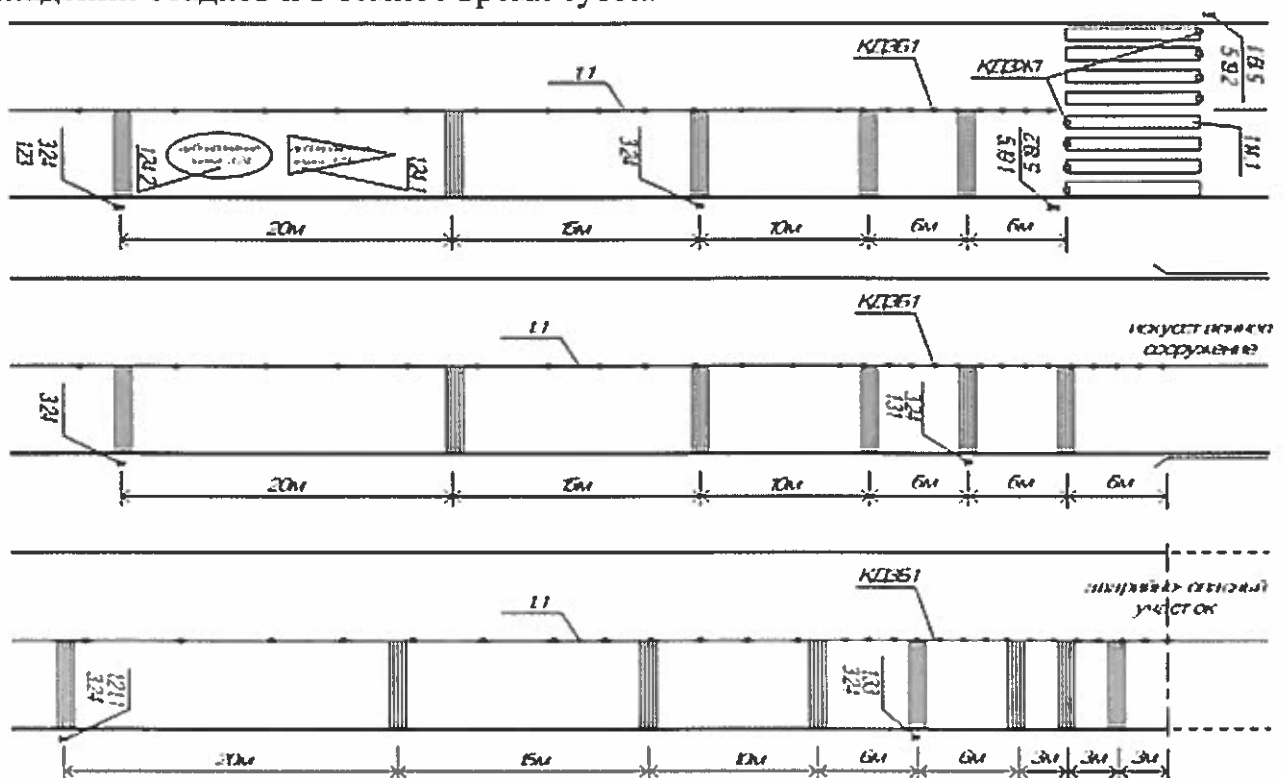
Рисунок 4.3 - Обустройство участков с поперечными световыми и световыми шумовыми полосами (пример)
