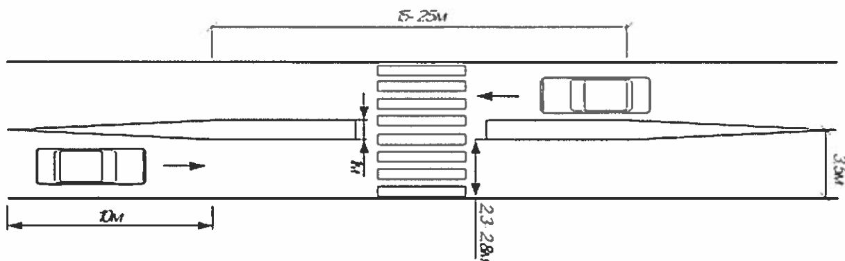
Рисунок 2.8 – Изменение эффективной ширины проезжей части (метод № 5)
