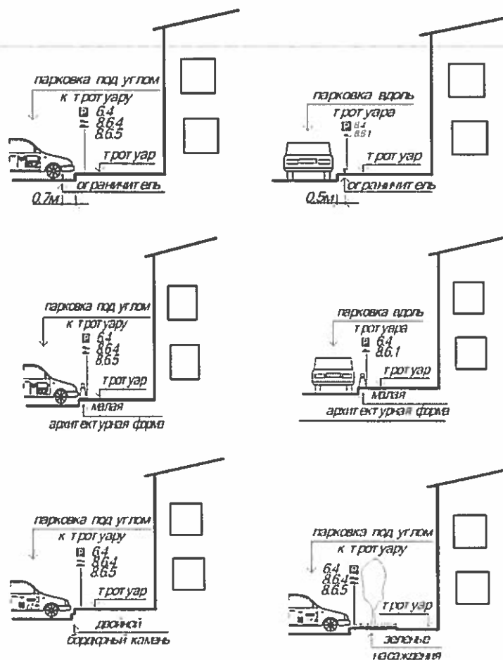
Рисунок 8.4 – Ограничение доступа автомобилей к тротуару при использовании
