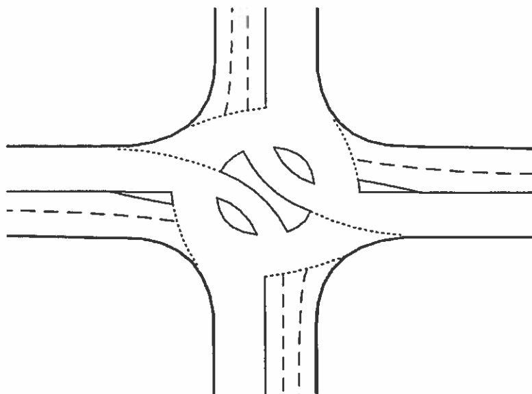
Рисунок 5.1 - Пересечение канализированного типа со сложной планировкой (Вариант №1)
