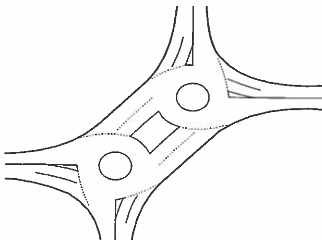
Рисунок 5.3 - Пересечение канализированного типа со сложной планировкой (Вариант №3)
