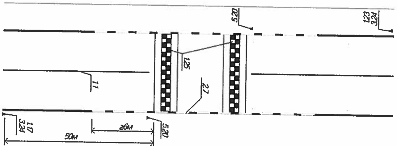
Рисунок 6.1 - Обустройство участков УДС с искусственными неровностями трапецевидного профиля
