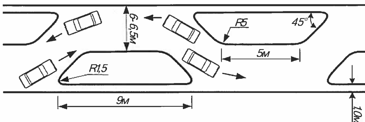
Рисунок 3.1 – Принципиальная схема организации зигзагообразного движения автомобилей посредством размещения трапецевидных направляющих островков
