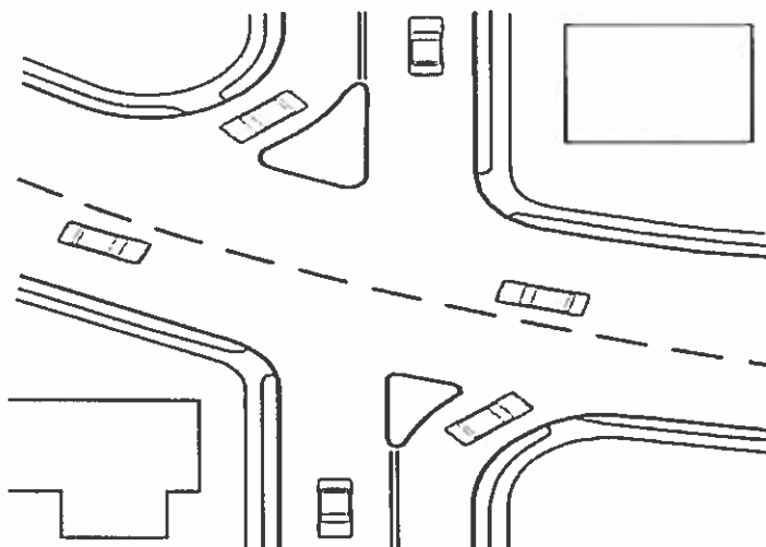
Рисунок 7.10 - Вариант обустройства для исключения сквозных проездов (пример № 3)
