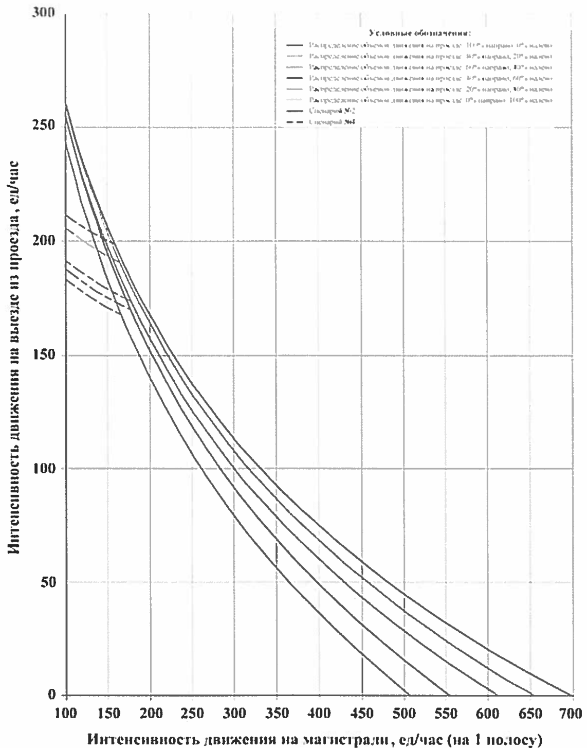
Рисунок 7.7 - Номограмма выбора максимального объема движения, приходящегося на один проезд при совместном движении пешеходов и автомобилей по территории проездов-проходов
