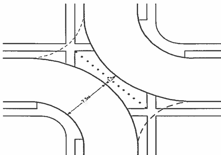
Рисунок 7.11 - Геометрические параметры диагональных перемычек
