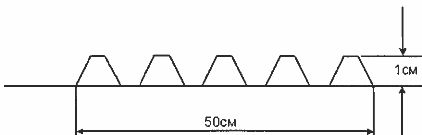
Рисунок 4.2 – Шумовые полосы из пластичных материалов
