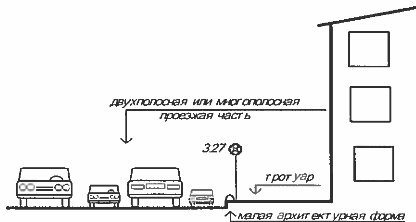
Рисунок 8.7 - Ограничение доступа автомобилей к тротуару с использованием малых архитектурных форм при наличии многополосной проезжей части дороги
