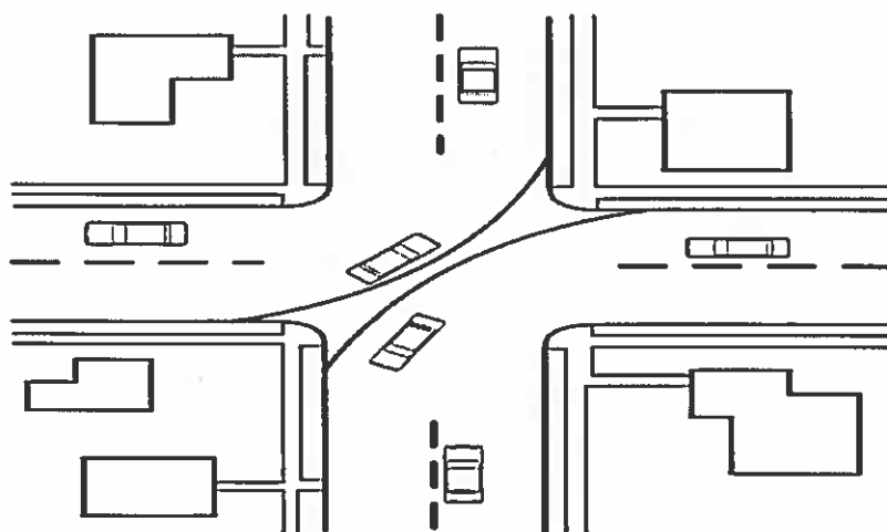
Рисунок 7.8 - Исключения сквозных проездов (Пример № 1)
