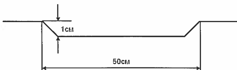
Рисунок 4.1 - Шумовые полосы, вырезанные на проезжей части
