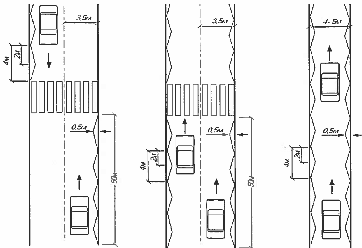
Рисунок 3.6 - Параметры зигзагообразной разметки
