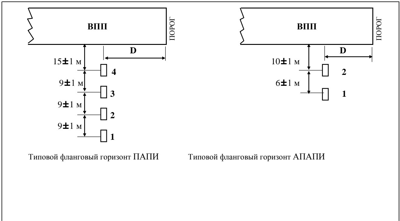
Рис. 5.22. Расположение систем ПАПИ и АПАПИ
