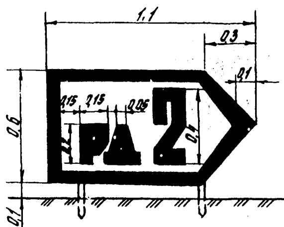
Рис. П.6.7. Знак РД
