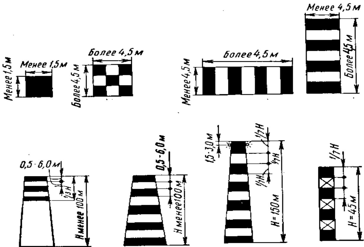
Рис. П.8.1. Примеры маркировки объектов
