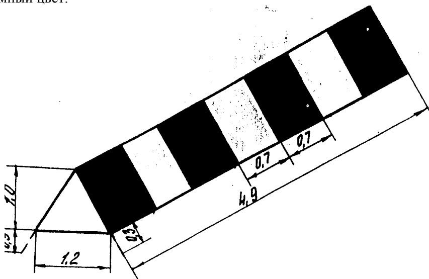
Рис. П.4.5. Входной маркер
