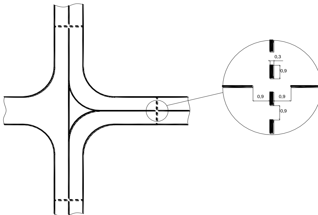
Рис. 5.3. Схема маркировки места пересечения РД
