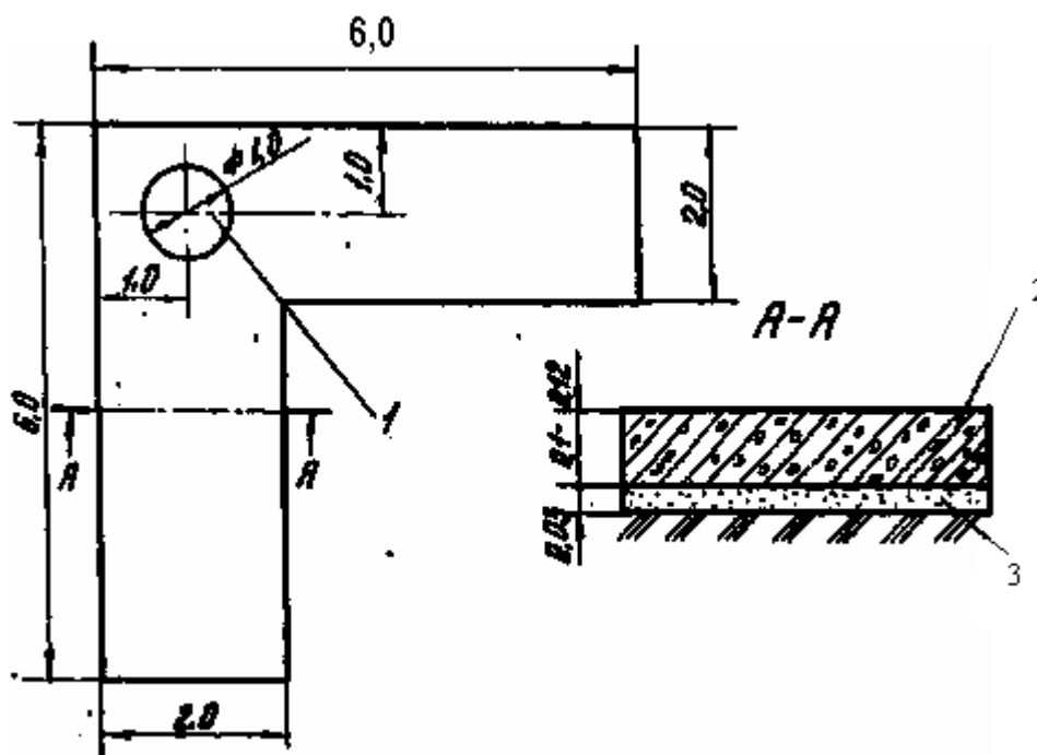
Рис. П.4.1. Угловой маркировочный знак
