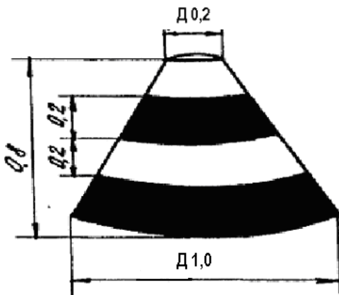
Рис. П.4.4 Пограничный маркер
