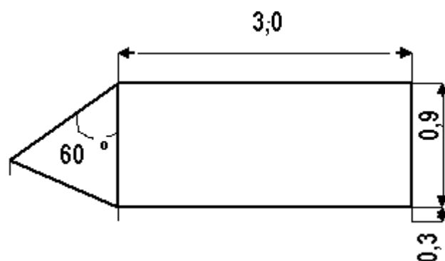
Рис. П.4.6. Маркер зоны приземления
