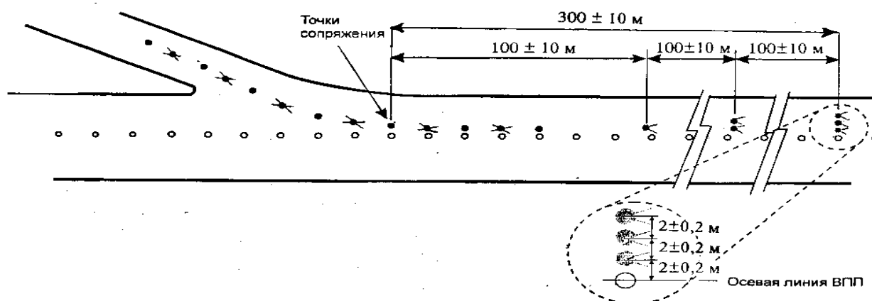
Рис. 5.21. Огни указателя РД быстрого схода с ВПП.
