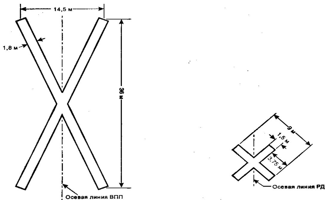
Рис. 5.7. Маркировка закрытых для движения ВПП и РД.
