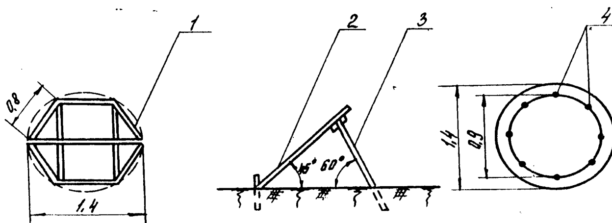
Рис. П.4.7. Маркер центра полосы
