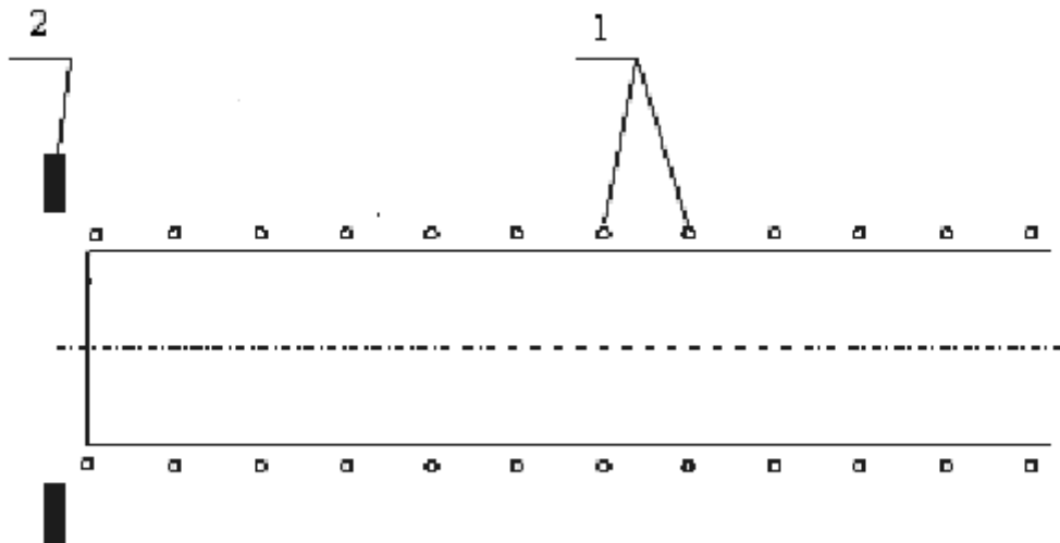
Рис. 5.29. Схема оборудования ГВПП класса Е маркерами: 1 – пограничный маркер; 2 – входной маркер.
