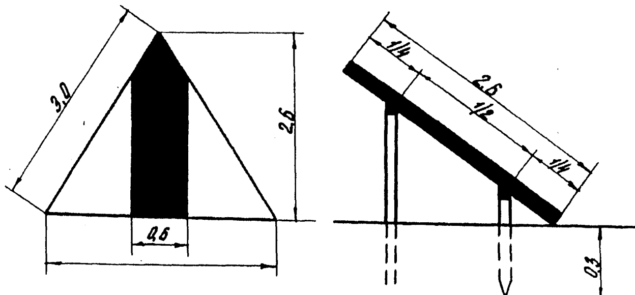
Рис. П.4.2 Маркер подхода
