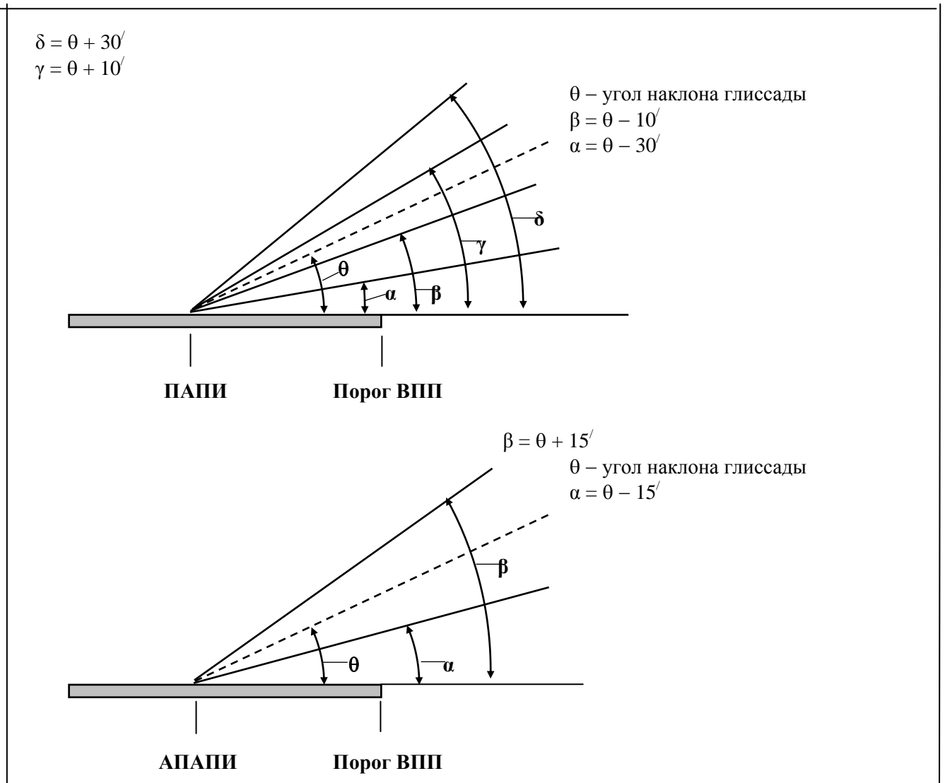
Рис. 5.23. Углы возвышения огней в системах ПАПИ и АПАПИ (для углов наклона глissады 2^{\circ} - 4^{\circ} )
