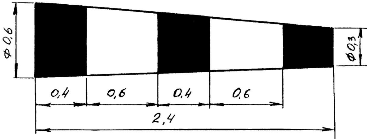
Рис. П.10.1. Конус-ветроуказатель
