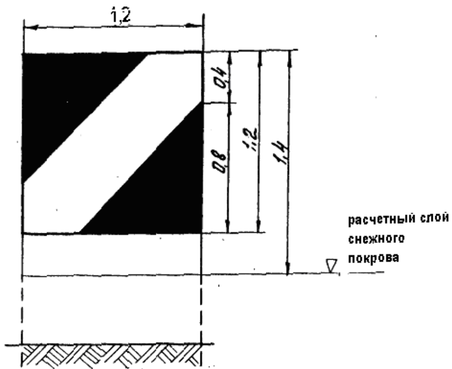
Рис. П.4.8. Маркер боковой границы
