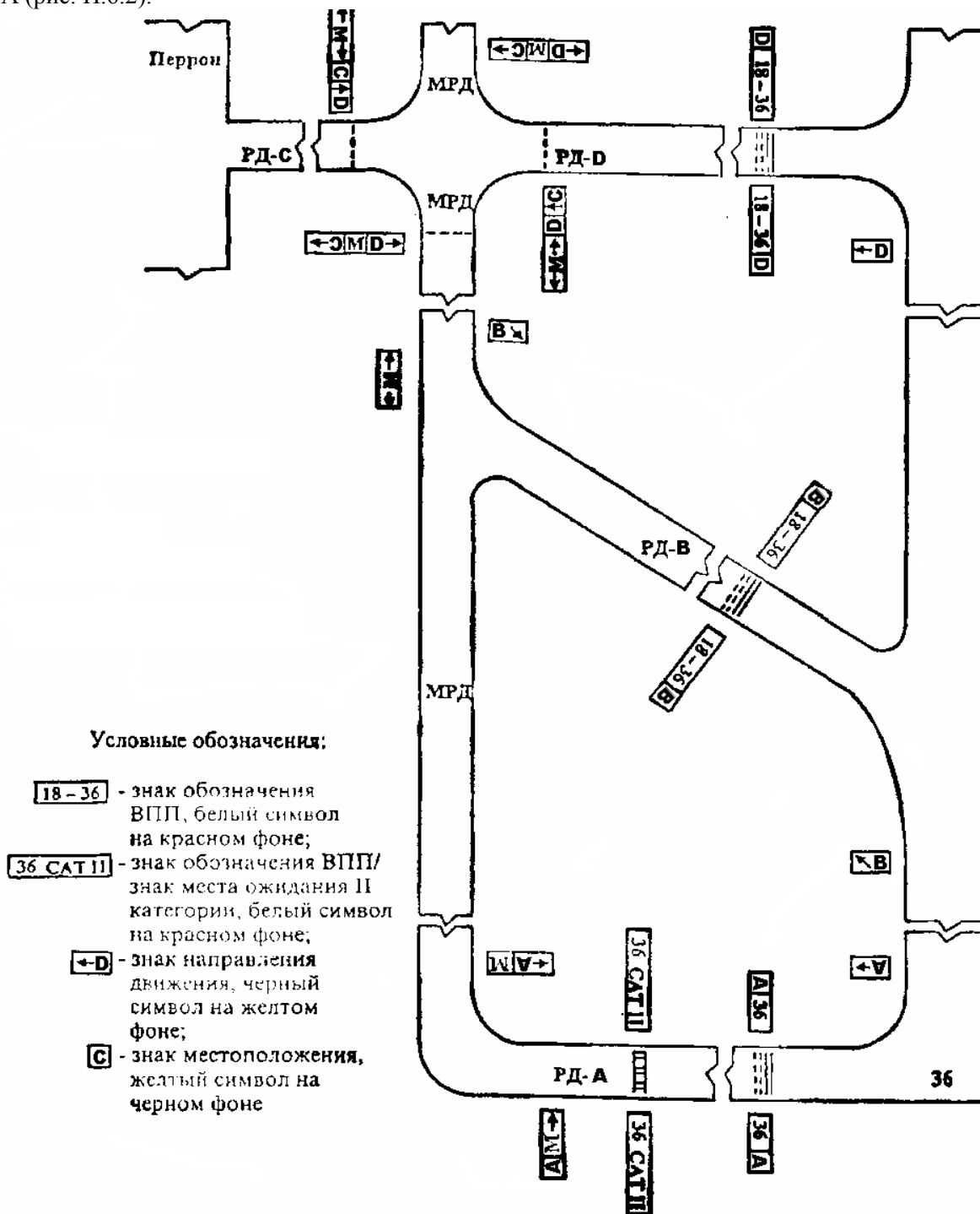
Рис. П.6.4. Пример расположения аэродромных знаков.
