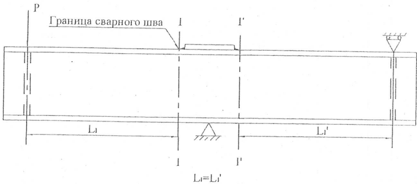
Рисунок А.6 Схема нагружения типового сварного образца (точка приложения пульсирующей нагрузки P может быть изменена в зависимости от конструкции стенда)
