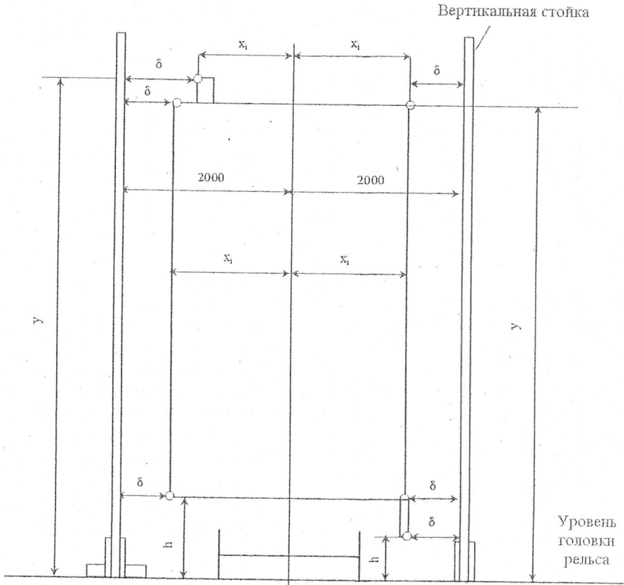
Рисунок А.1 Схема измерения габаритных размеров
