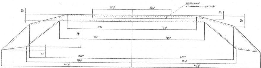
Рисунок А.15 Положение полоза токоприемника
