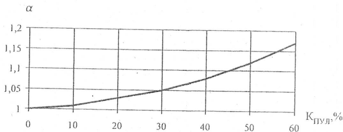
Рисунок А.8 График для определения эквивалентного коэффициента, учитывающего пульсацию тока
