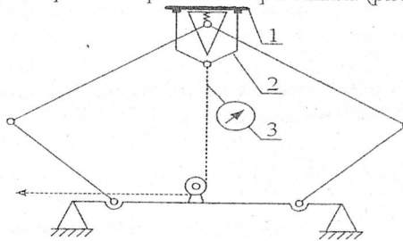
Рисунок А.18 Схема для определения аэродинамической характеристики токоприемников: 1 – отрезок контактного провода; 2 – рама; 3 – шнур
