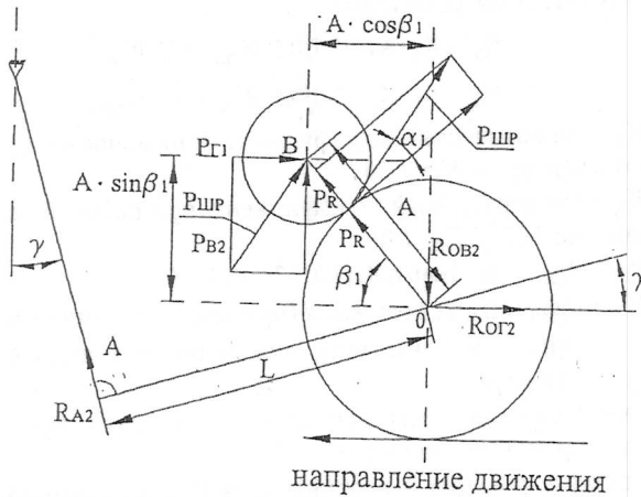
Рис. А.11. Схема нагружения опор редуктора в режиме тяги при движении тяговым электродвигателем вперед
