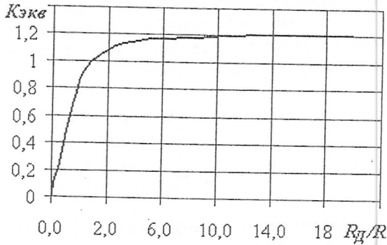
Рис. А.7. Графики для определения коэффициента учета внешних динамических нагрузок на якорные подшипники K_{ЭКВ}
