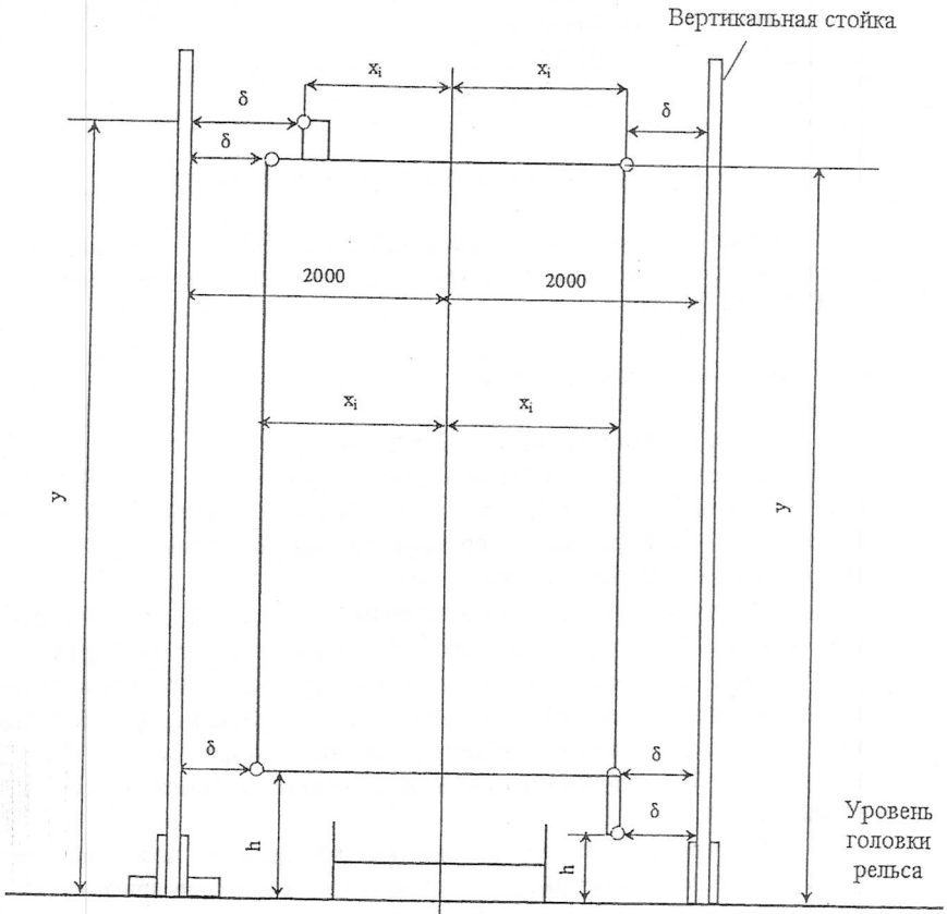
Рис. А.1. Схема измерения габаритных размеров
