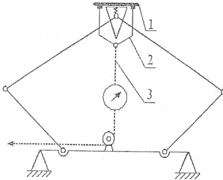
Рис. А.16. Схема для определения аэродинамической характеристики токоприемников: 1 – отрезок контактного провода; 2 – рама; 3 – шнур.
