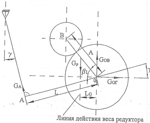
Рис. А.9. Схема нагружения опор весом тягового редуктора
