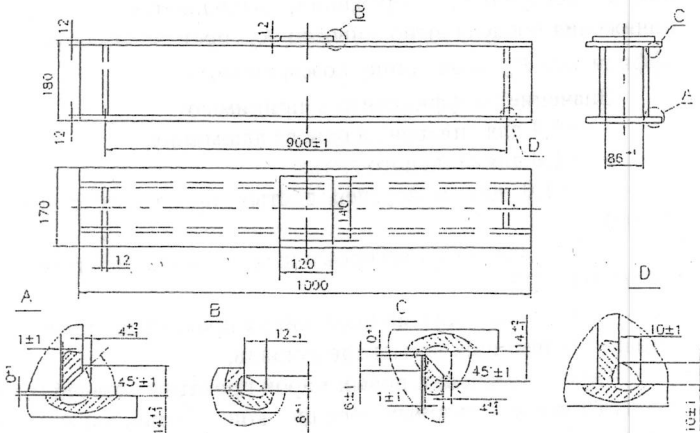
Рис. А.3. Типовой сварной образец
