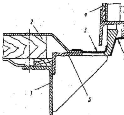
Рис.8.5. Заделка щелей порога дверного проема: 1 - продольная балка рамы вагона; 2 - пол; 3 - стеклоткань; 3 4 - створка двери; 5 - порог дверного проема
