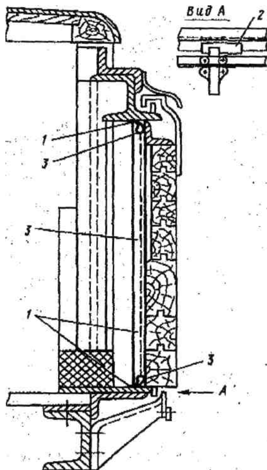
Рис. 8.3. заделка щелей в рабочей двери вагона бумагой:
